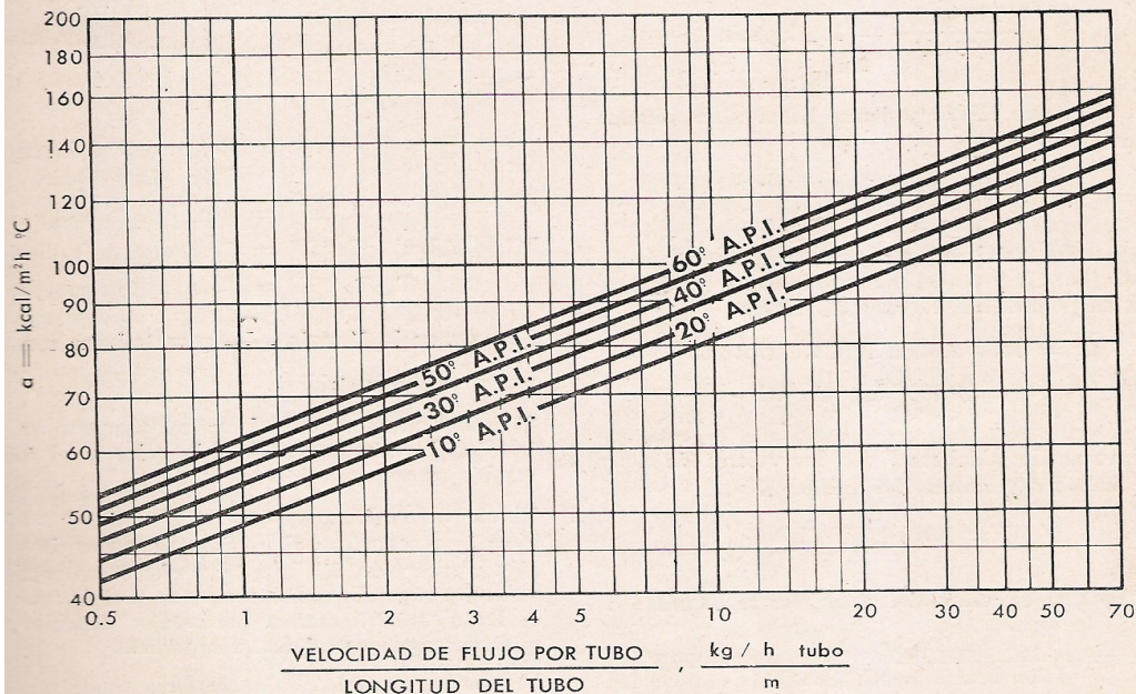
Gráfico 9: CONVECCION FORZADA DE PETROLEO CIRCULANDO DENTRO O FUERA DE TUBOS CON EL FLUJO PARALELO A ELLOS
