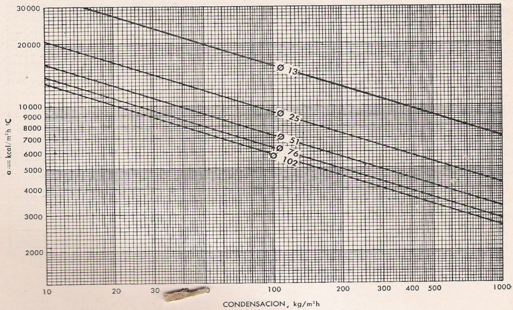
Gráfico 8: CONVECCION NATURAL DE VAPORES CONDENSANDOSE SOBRE TUBOS HORIZONTALES
