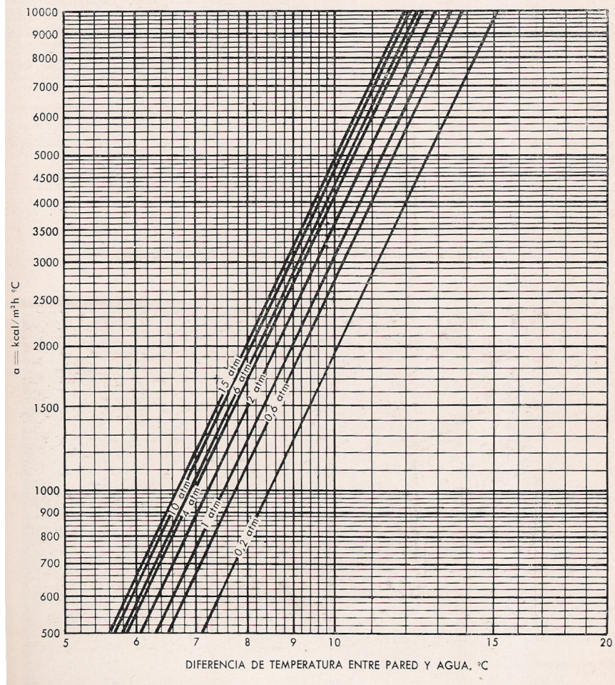
Gráfico 7: CONVECCION NATURAL DE AGUA HIRVIENDO SOBRE PLACAS PLANAS EN CUALQUIER POSICION
